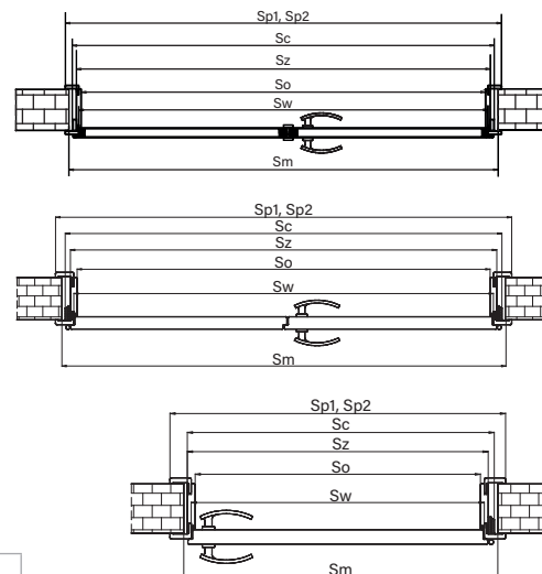
WYMIARY OŚCIEŻNICY REGULOWANEJ SW/S8 DO DRZWI JEDNOSKRZYDŁOWYCH
